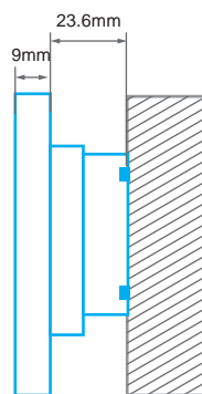
牆面安裝
