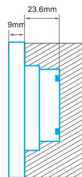
嵌入式安裝
